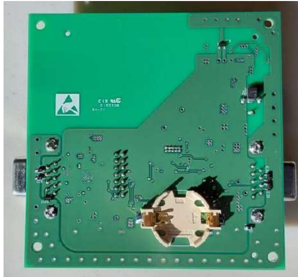
Placa de oximetria (SpO 2 ) desenvolvida na Contronic – vista inferior.
