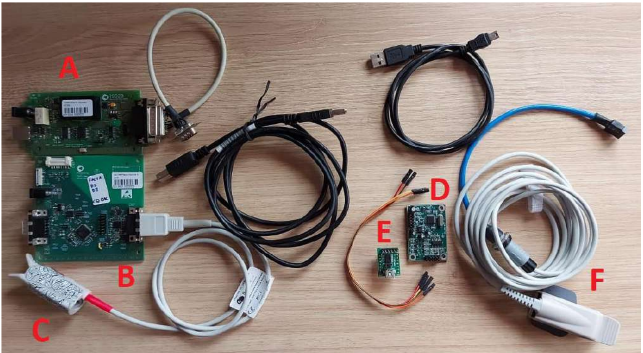
Setup usado durante o desenvolvimento e validação da placa de SpO 2 : A) placa ISO20; B) placa SpO 2 desenvolvida na Contronic; C) cabo de SpO 2 escolhido para o projeto; D) placa comercial de SpO 2 usada como base de comparação; E) interface UART/USB da placa comercial; F) sensor de SpO 2 da placa comercial.
