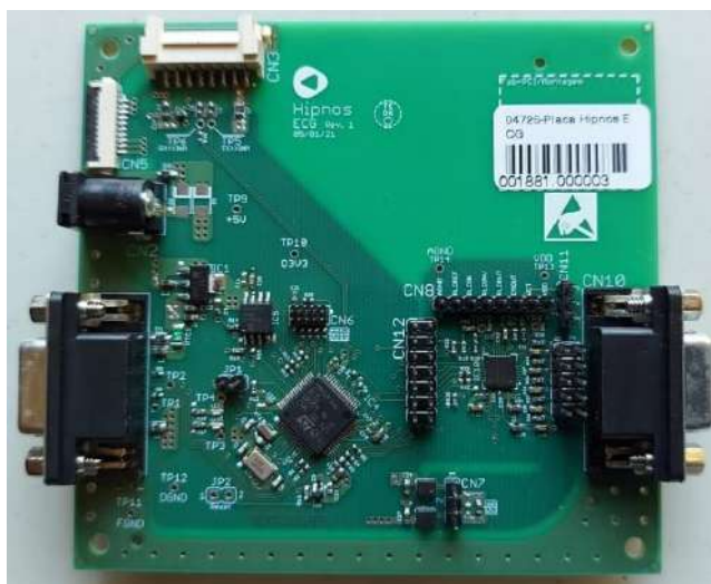
Placa de eletrocardiografia (ECG) desenvolvida na Contronic – vista superior.
