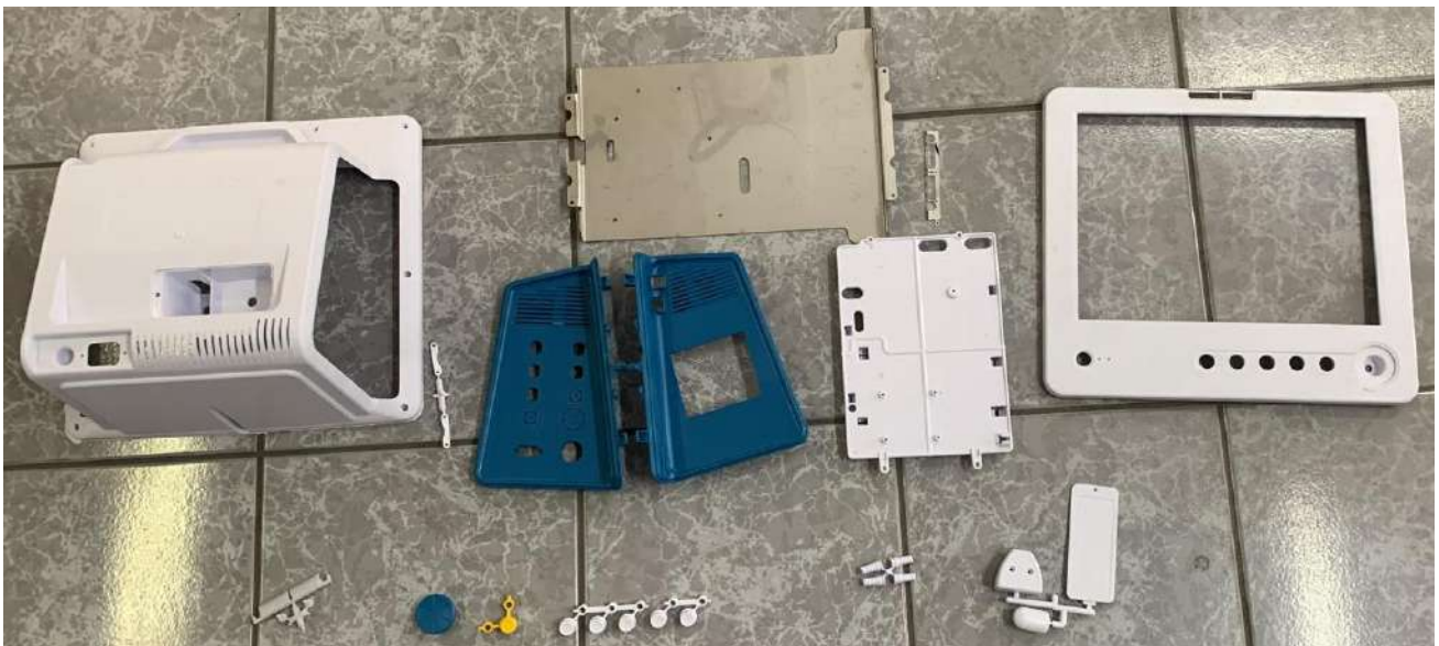
Conjunto de peças plásticas injetadas nas cores definitivas do produto e suporte metálico do display, material entregue pelo fornecedor apenas em novembro/22, após correções nos moldes.
